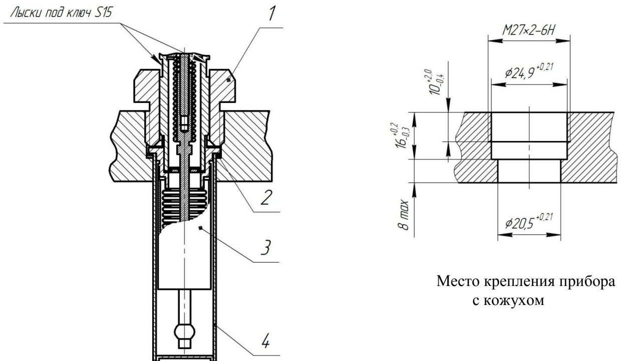
Рисунок А.3 – Крепление прибора без кожуха
